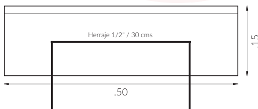
ALZADO LONGITUDINAL E:1/10
