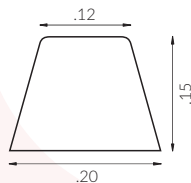
ALZADO TRANSVERSAL E:1/10
