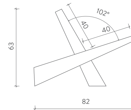
ALZADO LATERAL
