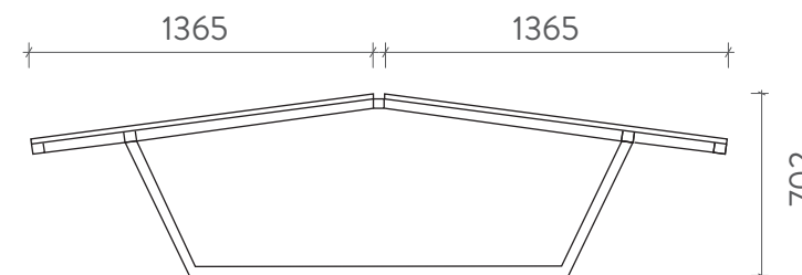
ALZADO LATERAL
