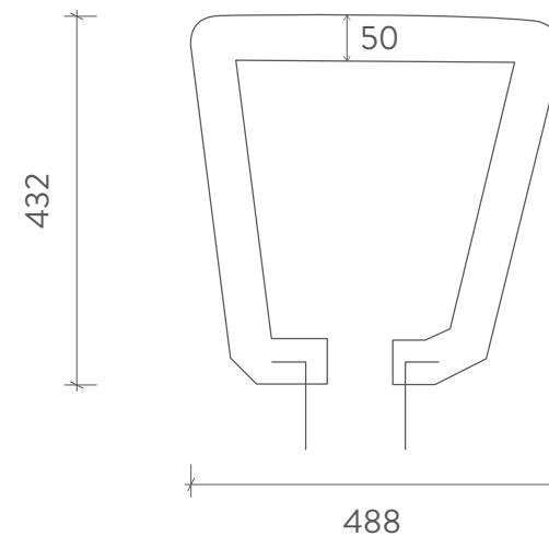
SECCIÓN TRANSVERSAL
