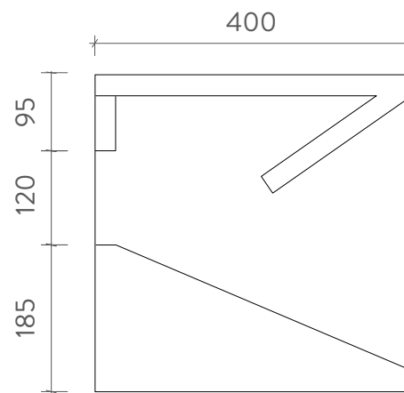
SECCIÓN TRANSVERSAL
