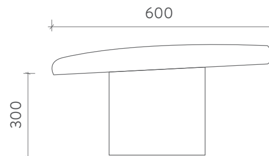
ALZADO LATERAL
