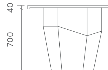
ALZADO FRONTAL
